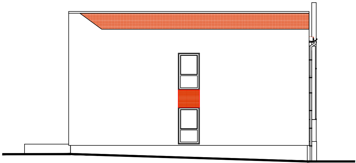
ELEWACJA BOCZNA
